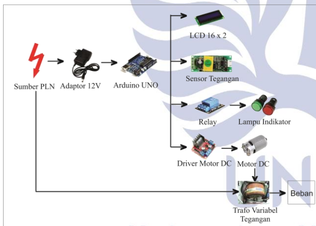
Gambar 11. Rancangan Sistem
