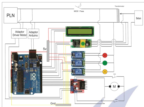
Gambar 14. Rangkaian pada Prototype Penstabil Tegangan
