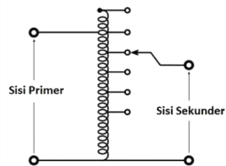
Gambar 1. Transformator Variabel Tegangan 1 fasa ( ( Sumber : Abdulrajak, 1985)
