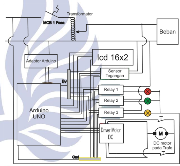
Gambar 2. Skema Rancangan
