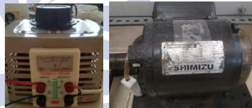
Gambar 23. Regulator tegangan dan Spesifikasi Motor Induksi 1 fasa 125W yang digunakan pengujian
