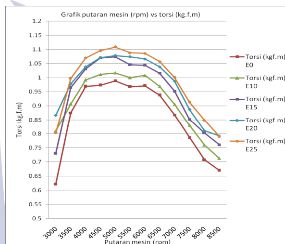
Gambar 3. Grafik Putaran Mesin Terhadap Torsi
