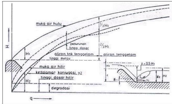
Gambar 3.2. Metode Perencanaan Kolam Loncat Air
