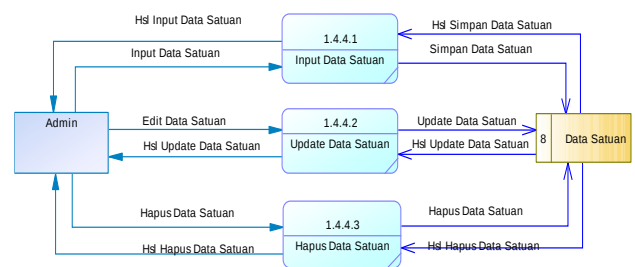
Gambar 4. DFD Level 3 Sistem Aplikasi Point Of Sale UD. Es Drop Cita Rasa Trenggalek
