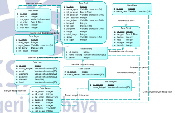
Gambar 5. CDM Sistem Aplikasi Point Of Sale UD. Es Drop Cita Rasa Trenggalek
