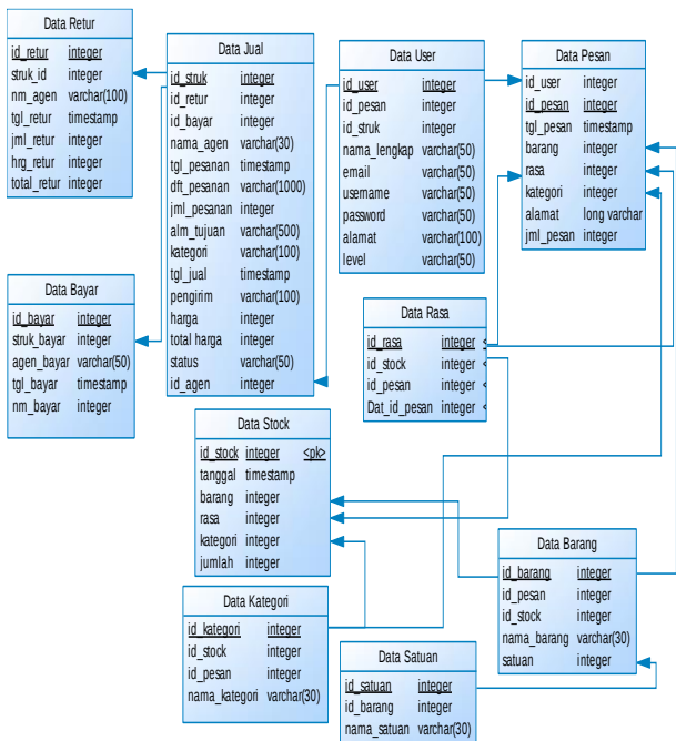
Gambar 6. PDM Sistem Aplikasi Point Of Sale UD. Es Drop Cita Rasa Trenggalek
