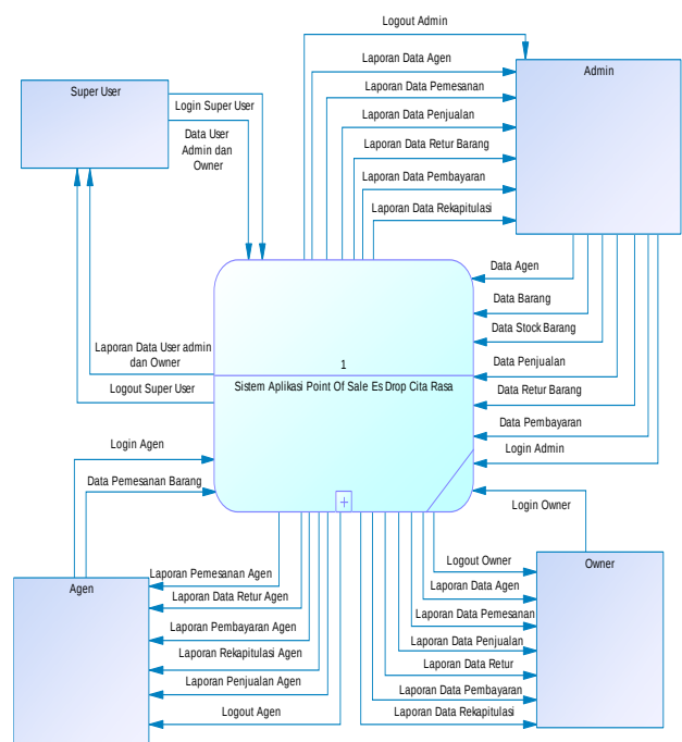
Gambar 1. DFD Level 0 (Diagram Konteks) Sistem Aplikasi Point Of Sale UD. Es Drop Cita Rasa Trenggalek
