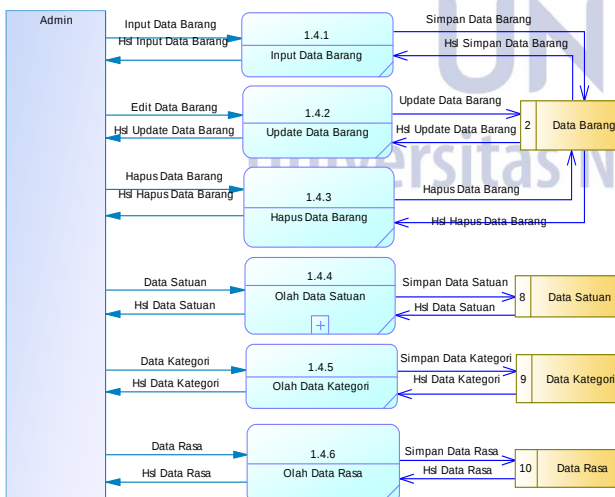
Gambar 3. DFD Level 2 Sistem Aplikasi Point Of Sale UD. Es Drop Cita Rasa Trenggalek
