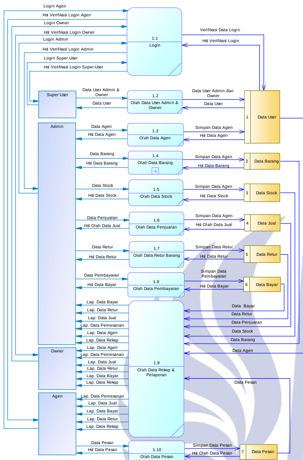
Gambar 2. DFD Level 1 Sistem Aplikasi Point Of Sale UD. Es Drop Cita Rasa Trenggalek
