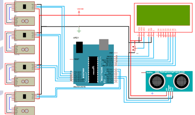
Gambar 3.5 Rangkaian Keseluruhan Alat Yang Dibuat (Sumber : Data Primer, 2017)
