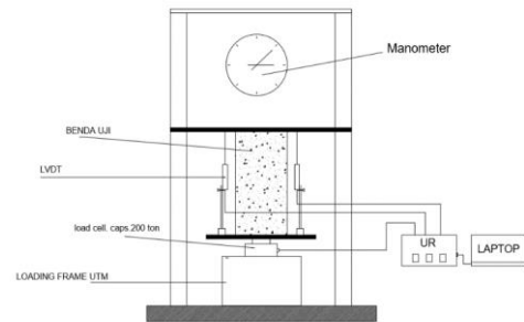
Gambar 3. Set up pengujian
