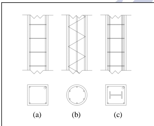
Gambar 1. Jenis Kolom berdasarkan jenis tulangan
