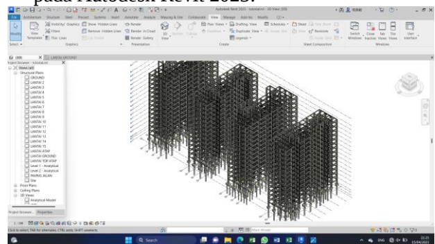
Gambar 10. Pemodelan 3D Struktur Balok
